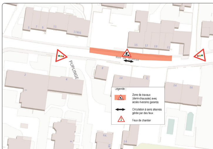
Principe de fonctionnement d'une étape de chantier
